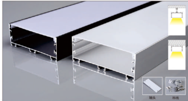
PG56X 产品参数 10035 尺寸: Lx100x35mm 表面: 氧化铝本色/喷漆 (黑色/白色) PC罩: 乳白 适用: 92MM软灯带/硬灯条
