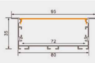
PG70X 产品参数 8035带边 尺寸: Lx95x35mm 表面: 氧化铝本色/喷漆 (黑色/白色) PC罩: 乳白 适用: 72MM软灯带/硬灯条
