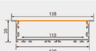
PG62X 产品参数 12035带边 尺寸: Lx135x35mm 表面: 氧化铝本色/喷漆 (黑色/白色) PC罩: 乳白 适用: 110MM软灯带/硬灯条
