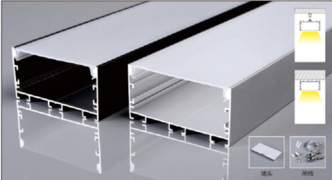
PG88X 产品参数 7035 尺寸: Lx70x35mm 表面: 氧化铝本色/喷漆 (黑色/白色) PC罩: 乳白 适用: 62MM软灯带/硬灯条
