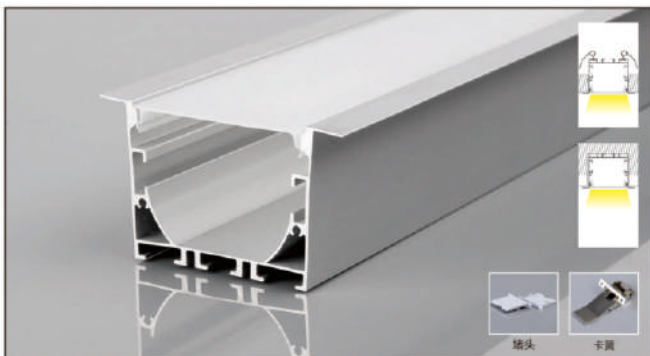
PG10X 产品参数 5040带边 尺寸: Lx66x40mm 表面: 氧化铝本色/喷漆 (黑色/白色) PC罩: 乳白/黑色/亚克力磨砂可选 适用: 26MM软灯带/硬灯条
