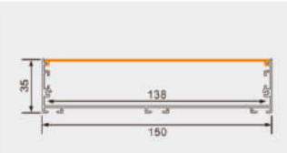
PR15035X 产品参数 15035 尺寸: Lx150x35mm 表面: 氧化铝本色/喷漆 (黑色/白色) PC罩: 乳白/黑色/亚克力磨砂可选 适用: 138MM软灯带/硬灯条
