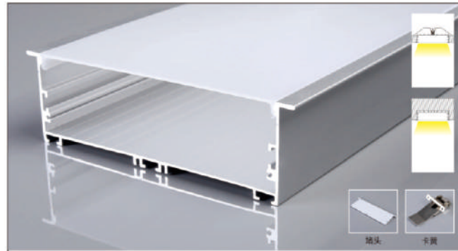
PG117X 产品参数 15050带边 尺寸: Lx166x50mm 表面: 氧化铝本色/喷漆 (黑色/白色) PC罩: 乳白 适用: 140MM软灯带/硬灯条
