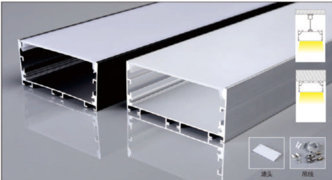
PG29X 产品参数 7535 尺寸: Lx80x35mm 表面: 氧化铝本色/喷漆 (黑色/白色) PC罩: 乳白 适用: 72MM软灯带/硬灯条
