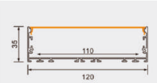
PG61X 产品参数 12035 尺寸: Lx120x35mm 表面: 氧化铝本色/喷漆 (黑色/白色) PC罩: 乳白 适用: 110MM软灯带/硬灯条
