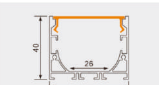
PG02X 产品参数 5040 尺寸: Lx50x40mm 表面: 氧化铝本色/喷漆 (黑色/白色) PC罩: 乳白/黑色/亚克力磨砂可选 适用: 26MM软灯带/硬灯条
