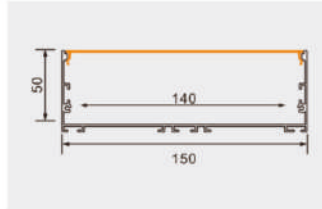
PG116X 产品参数 15050 尺寸: Lx150x50mm 表面: 氧化铝本色/喷漆 (黑色/白色) PC罩: 乳白 适用: 140MM软灯带/硬灯条
