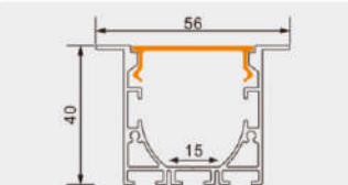
PG09X 产品参数 4040带边 尺寸: Lx56x40mm 表面: 氧化铝本色/喷漆 (黑色/白色) PC罩: 乳白/黑色/亚克力磨砂可选 适用: 15MM软灯带/硬灯条
