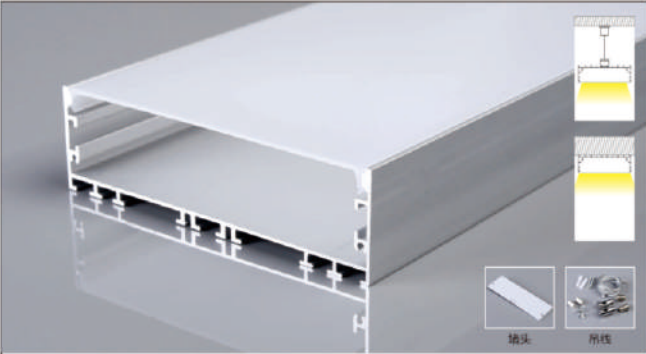
PG61X 产品参数 12035 尺寸: Lx120x35mm 表面: 氧化铝本色/喷漆 (黑色/白色) PC罩: 乳白 适用: 110MM软灯带/硬灯条
