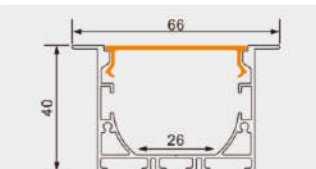
PG10X 产品参数 5040带边 尺寸: Lx66x40mm 表面: 氧化铝本色/喷漆 (黑色/白色) PC罩: 乳白/黑色/亚克力磨砂可选 适用: 26MM软灯带/硬灯条
