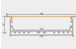
PG15X 产品参数 15040带边 尺寸: Lx166x40mm 表面: 氧化铝本色/喷漆 (黑色/白色) PC罩: 乳白/黑色/亚克力磨砂可选 适用: 125MM软灯带/硬灯条
