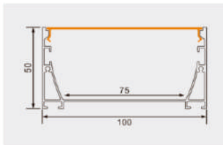
PG82X 产品参数 10050 尺寸: Lx100x50mm 表面: 氧化铝本色/喷漆 (黑色/白色) PC罩: 乳白/黑色/亚克力磨砂可选 适用: 75MM软灯带/硬灯条
