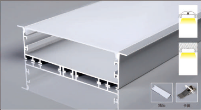
PG62X 产品参数 12035带边 尺寸: Lx135x35mm 表面: 氧化铝本色/喷漆 (黑色/白色) PC罩: 乳白 适用: 110MM软灯带/硬灯条
