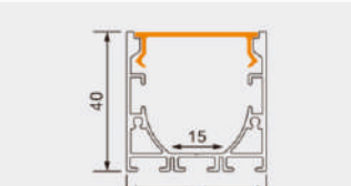
PG01X 产品参数 4040 尺寸: Lx40x40mm 表面: 氧化铝本色/喷漆 (黑色/白色) PC罩: 乳白/黑色/亚克力磨砂可选 适用: 15MM软灯带/硬灯条
