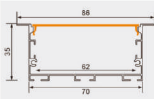
PG83X 产品参数 7035带边 尺寸: Lx86x35mm 表面: 氧化铝本色/喷漆 (黑色/白色) PC罩: 乳白 适用: 62MM软灯带/硬灯条
