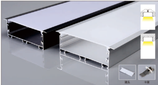
PG158X 产品参数 9035带边 尺寸: Lx116x35mm 表面: 氧化铝本色/喷漆 (黑色/白色) PC罩: 乳白 适用: 92MM软灯带/硬灯条
