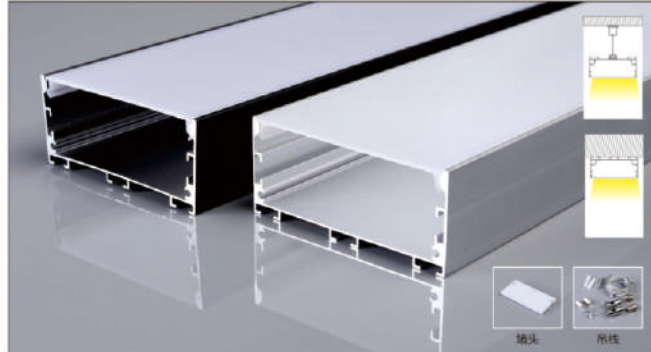
PG69X 产品参数 8035 尺寸: Lx80x35mm 表面: 氧化铝本色/喷漆 (黑色/白色) PC罩: 乳白 适用: 72MM软灯带/硬灯条
