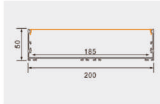
PG118X 产品参数 20050 尺寸: Lx200x50mm 表面: 氧化铝本色/喷漆 (黑色/白色) PC罩: 乳白 适用: 185MM软灯带/硬灯条
