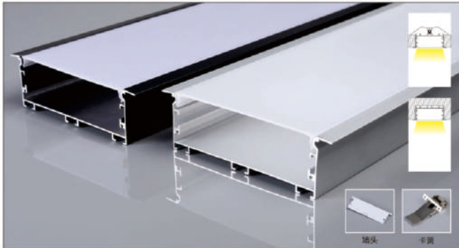
PG57X 产品参数 10035带边 尺寸: Lx116x35mm 表面: 氧化铝本色/喷漆 (黑色/白色) PC罩: 乳白 适用: 92MM软灯带/硬灯条
