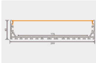
PG08X 产品参数 20040 尺寸: Lx200x40mm 表面: 氧化铝本色/喷漆 (黑色/白色) PC罩: 乳白/黑色/亚克力磨砂可选 适用: 175MM软灯带/硬灯条
