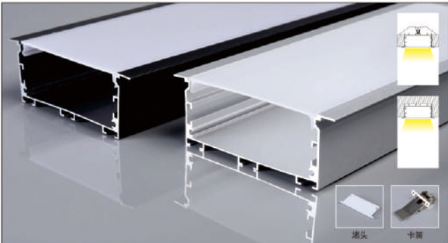
PG30X 产品参数 7535带边 尺寸: Lx95x35mm 表面: 氧化铝本色/喷漆 (黑色/白色) PC罩: 乳白 适用: 72MM软灯带/硬灯条
