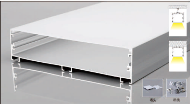
PR15035X 产品参数 15035 尺寸: Lx150x35mm 表面: 氧化铝本色/喷漆 (黑色/白色) PC罩: 乳白/黑色/亚克力磨砂可选 适用: 138MM软灯带/硬灯条
