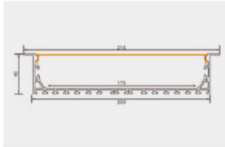
PG16X 产品参数 20040带边 尺寸: Lx216x40mm 表面: 氧化铝本色/喷漆 (黑色/白色) PC罩: 乳白/黑色/亚克力磨砂可选 适用: 175MM软灯带/硬灯条
