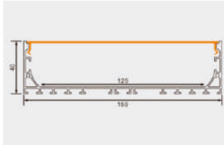
PG07X 产品参数 15040 尺寸: Lx150x40mm 表面: 氧化铝本色/喷漆 (黑色/白色) PC罩: 乳白/黑色/亚克力磨砂可选 适用: 125MM软灯带/硬灯条
