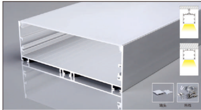
PG07X 产品参数 15040 尺寸: Lx150x40mm 表面: 氧化铝本色/喷漆 (黑色/白色) PC罩: 乳白/黑色/亚克力磨砂可选 适用: 125MM软灯带/硬灯条
