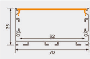
PG88X 产品参数 7035 尺寸: Lx70x35mm 表面: 氧化铝本色/喷漆 (黑色/白色) PC罩: 乳白 适用: 62MM软灯带/硬灯条
