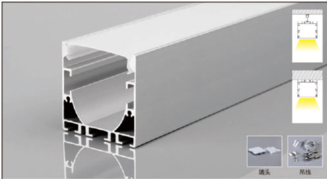
PG01X 产品参数 4040 尺寸: Lx40x40mm 表面: 氧化铝本色/喷漆 (黑色/白色) PC罩: 乳白/黑色/亚克力磨砂可选 适用: 15MM软灯带/硬灯条
