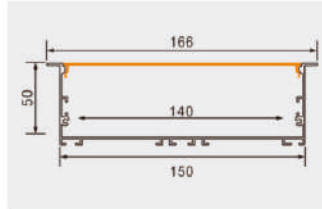
PG117X 产品参数 15050带边 尺寸: Lx166x50mm 表面: 氧化铝本色/喷漆 (黑色/白色) PC罩: 乳白 适用: 140MM软灯带/硬灯条
