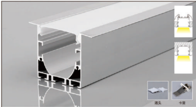
PG09X 产品参数 4040带边 尺寸: Lx56x40mm 表面: 氧化铝本色/喷漆 (黑色/白色) PC罩: 乳白/黑色/亚克力磨砂可选 适用: 15MM软灯带/硬灯条
