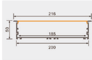
PG119X 产品参数 20050带边 尺寸: Lx216x50mm 表面: 氧化铝本色/喷漆 (黑色/白色) PC罩: 乳白 适用: 185MM软灯带/硬灯条
