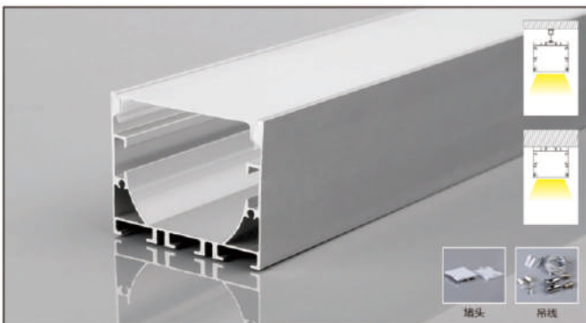
PG02X 产品参数 5040 尺寸: Lx50x40mm 表面: 氧化铝本色/喷漆 (黑色/白色) PC罩: 乳白/黑色/亚克力磨砂可选 适用: 26MM软灯带/硬灯条
