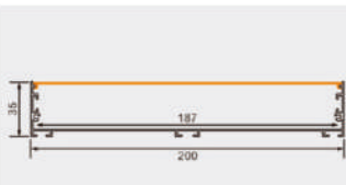
PR20035X 产品参数 20035 尺寸: Lx200x35mm 表面: 氧化铝本色/喷漆 (黑色/白色) PC罩: 乳白/黑色/亚克力磨砂可选 适用: 187MM软灯带/硬灯条
