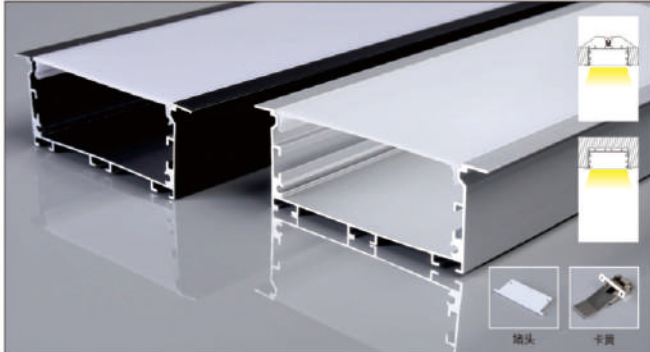
PG70X 产品参数 8035带边 尺寸: Lx95x35mm 表面: 氧化铝本色/喷漆 (黑色/白色) PC罩: 乳白 适用: 72MM软灯带/硬灯条
