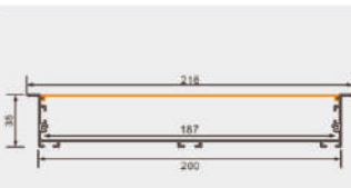
PR20035DBX 产品参数 20035带边 尺寸: Lx216x35mm 表面: 氧化铝本色/喷漆 (黑色/白色) PC罩: 乳白/黑色/亚克力磨砂可选 适用: 187MM软灯带/硬灯条
