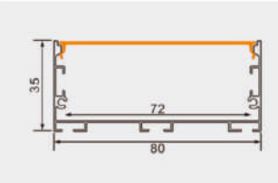
PG69X 产品参数 8035 尺寸: Lx80x35mm 表面: 氧化铝本色/喷漆 (黑色/白色) PC罩: 乳白 适用: 72MM软灯带/硬灯条
