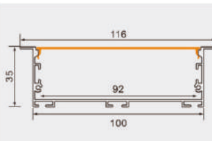
PG57X 产品参数 10035带边 尺寸: Lx116x35mm 表面: 氧化铝本色/喷漆 (黑色/白色) PC罩: 乳白 适用: 92MM软灯带/硬灯条
