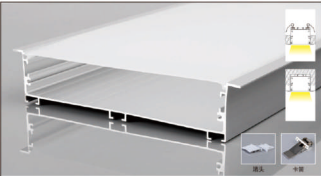
PR15035DBX 产品参数 15035带边 尺寸: Lx166x35mm 表面: 氧化铝本色/喷漆 (黑色/白色) PC罩: 乳白/黑色/亚克力磨砂可选 适用: 138MM软灯带/硬灯条
