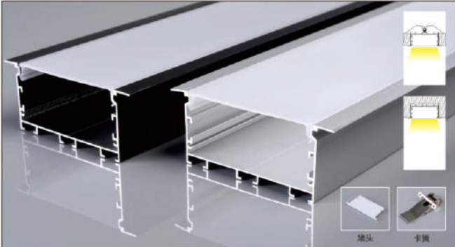
PG83X 产品参数 7035带边 尺寸: Lx86x35mm 表面: 氧化铝本色/喷漆 (黑色/白色) PC罩: 乳白 适用: 62MM软灯带/硬灯条
