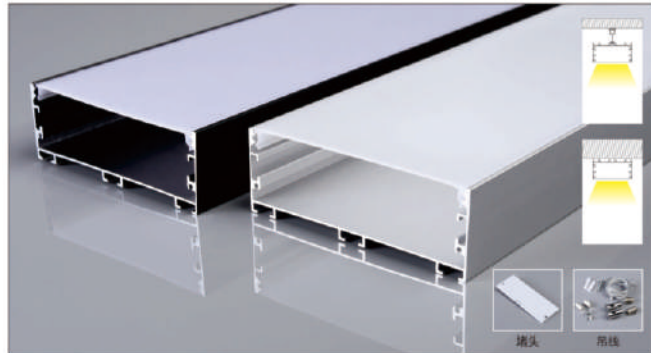
PG157X 产品参数 9035 尺寸: Lx100x35mm 表面: 氧化铝本色/喷漆 (黑色/白色) PC罩: 乳白 适用: 92MM软灯带/硬灯条
