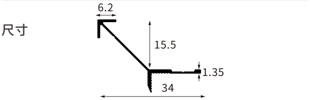
型号 AL-QB-1506A-15厘海棠阳角
