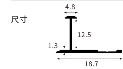
型号 AL-QB-1202A-12厘收口线
