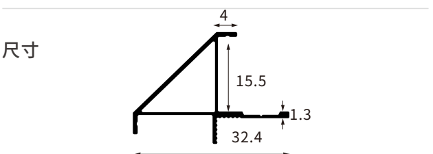
型号 AL-QB-1508A-15厘阴角线
