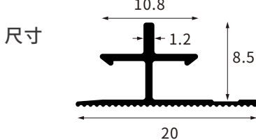
型号 AL-QB-0811A-8厘顶线
