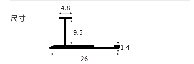
型号 AL-QB-0902A-9厘收口线
