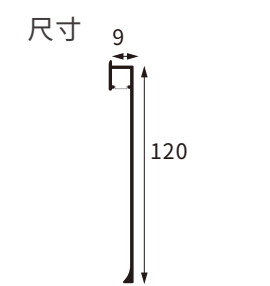
型号 AL-TJX-02H
