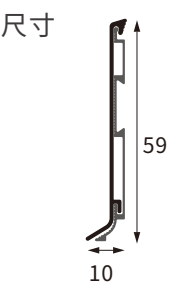
型号 AL-TJX-03D
