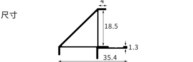
型号 AL-QB-1808A-18厘阴角线
