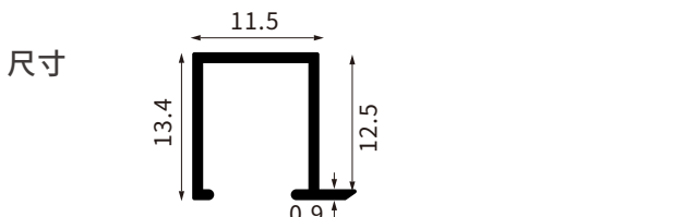
型号 AL-QB-1211A-12厘平缝线
