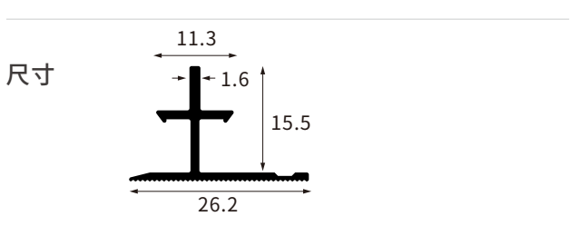
型号 AL-QB-1510A-15厘顶线
