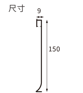
型号 AL-TJX-03H
