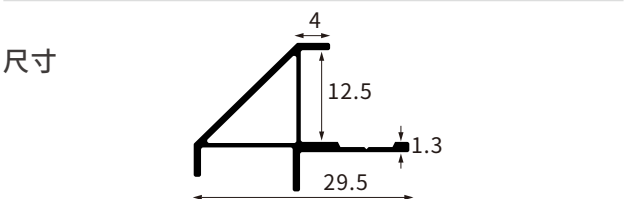
型号 AL-QB-1208A-12厘阴角线
