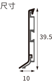
型号 AL-TJX-01D
