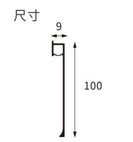
型号 AL-TJX-01H
