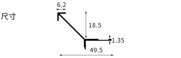
型号 AL-QB-1806A-18厘海棠阳角
