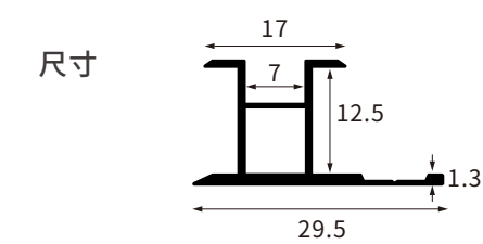
型号 AL-QB-1204A-12厘圆阳角
