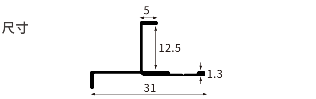
型号 AL-QB-1207A-12厘斜阳角
