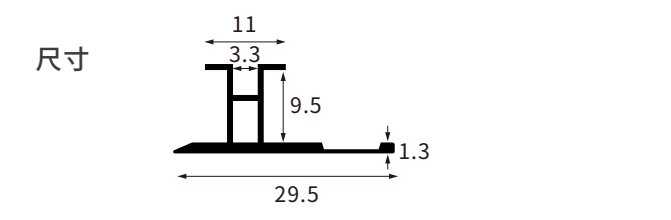
型号 AL-QB-0904A-9厘圆阳角
