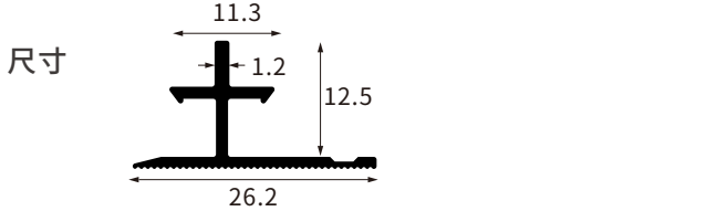
型号 AL-QB-1210A-12厘顶线
