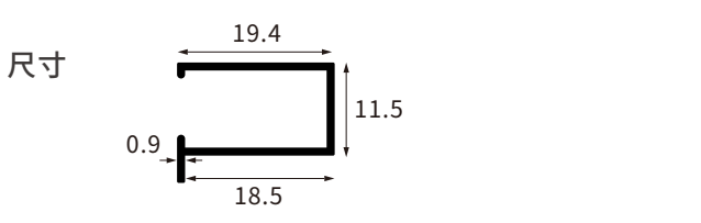
型号 AL-QB-1811A-18厘平缝线
