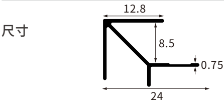
型号 AL-QB-0807A-8厘海棠阳角
