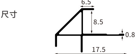
型号 AL-QB-0809A-8厘阴角线
