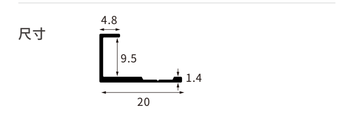
型号 AL-QB-0903A-9厘腰线
