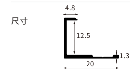
型号 AL-QB-1203A-12厘腰线
