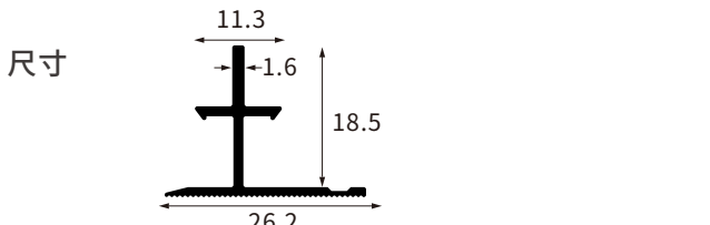
型号 AL-QB-1810A-18厘顶线
