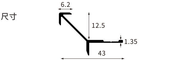
型号 AL-QB-1206A-12厘海棠阳角
