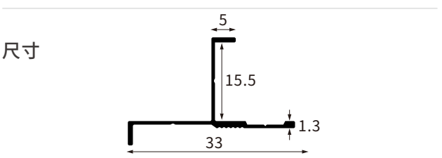
型号 AL-QB-1507A-15厘斜阳角
