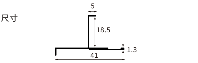
型号 AL-QB-1807A-18厘斜阳角
