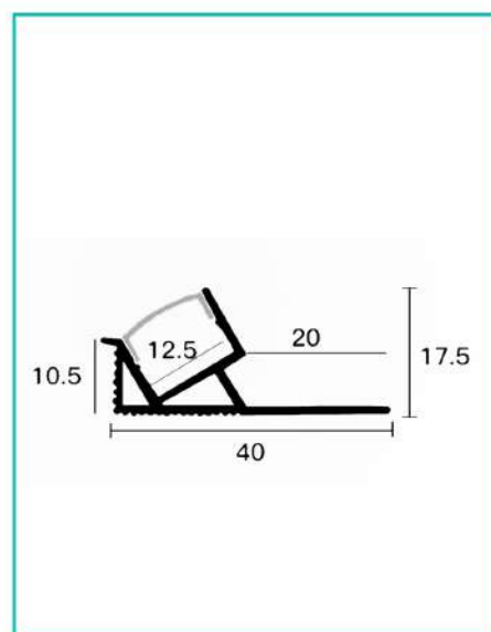
平装38度图纸
