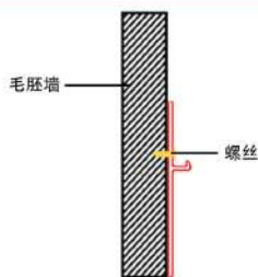
1-打螺丝固定踢脚线
