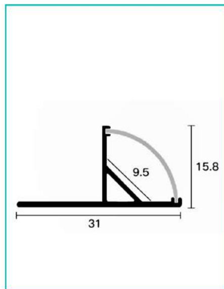
单边45度款图纸
