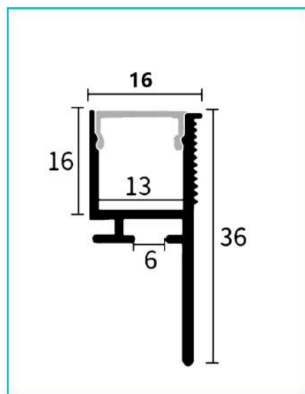
竖装向上款图纸
