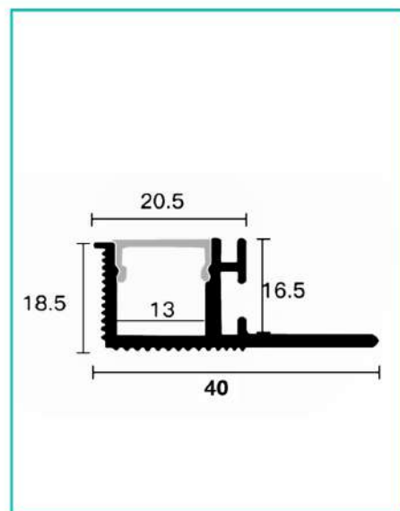
平装向上款图纸
