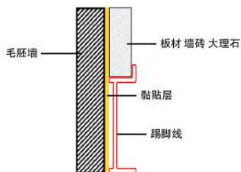
2-安装上踢脚线
